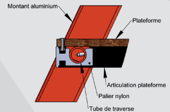
Coupe de l'articulation de plateforme et porte-outils avec paliers
